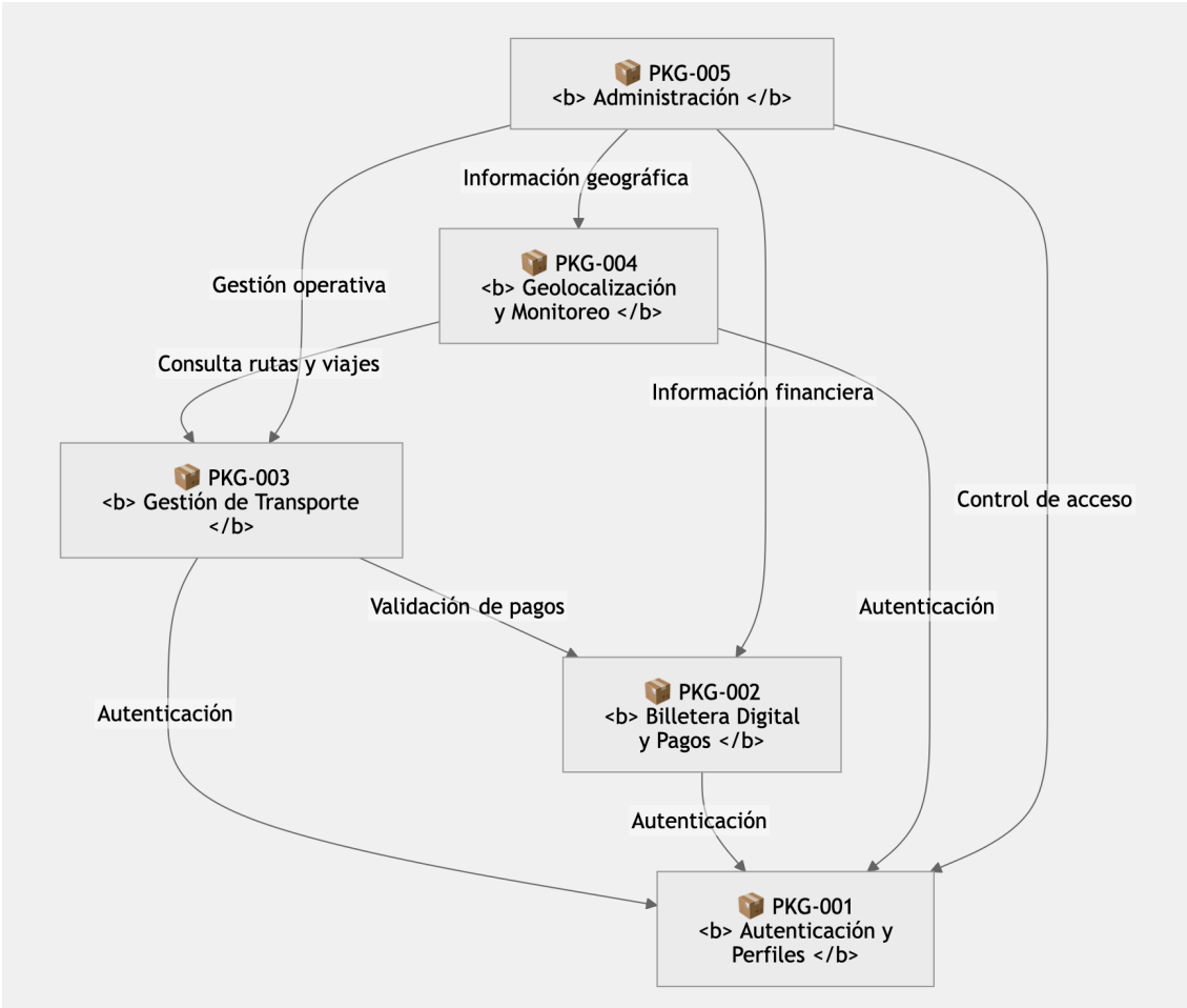
Diagrama UML agrupando módulos
